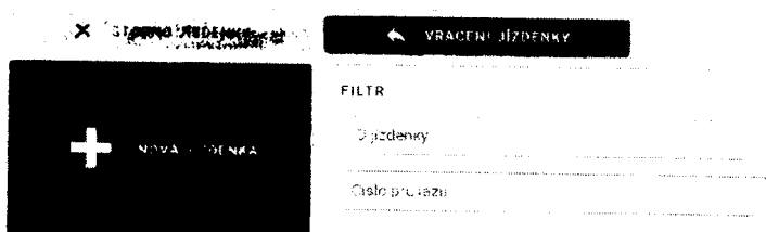
Obrázek 6 - Nová jízdenka
