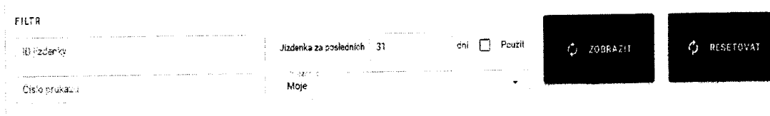
Obrázek 10 - Ovládání filtrování
