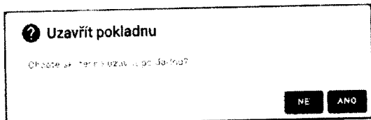
Obrázek 4 - Uzavřít pokladnu
